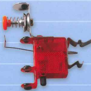
ESJ-2711 12V (Pin) ESJ-2712 24V (Pin)
